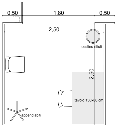
pianta
