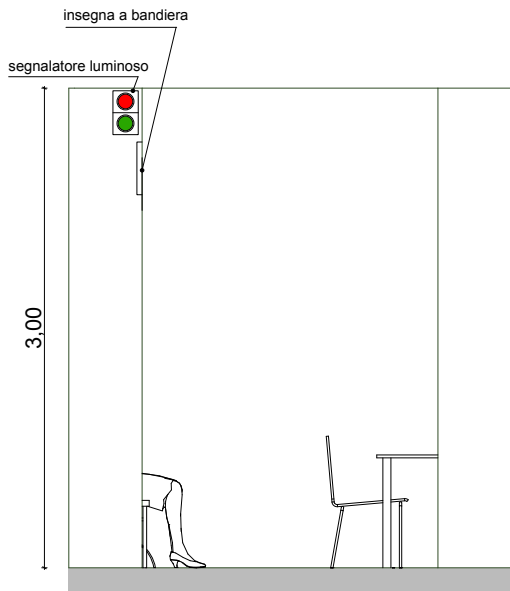
prospetto
